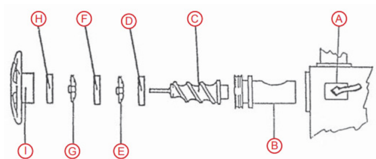
Obr. 2 Rozebírka dvousložení neodnímatelná
